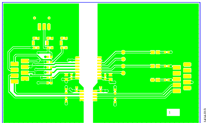
Figure 16. Top Layer
