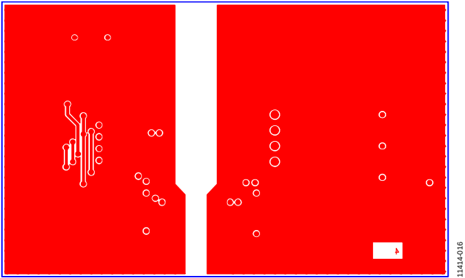
Figure 19. Bottom Layer
