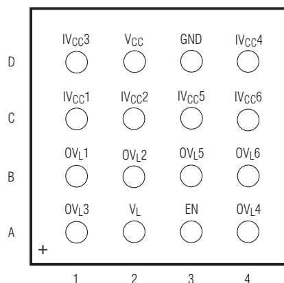
4 X 4 UCSP
