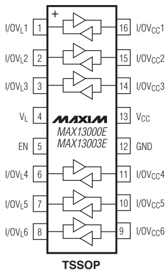
TSSOP
