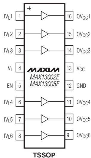
TSSOP
