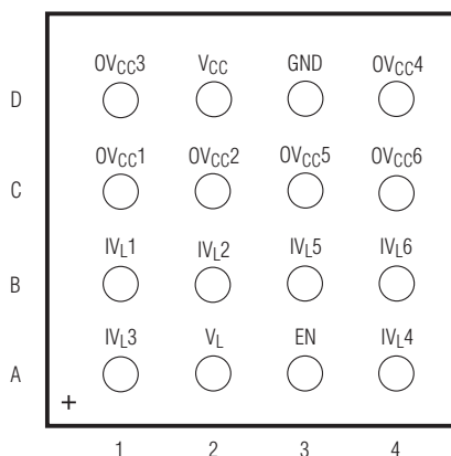
4 X 4 UCSP
