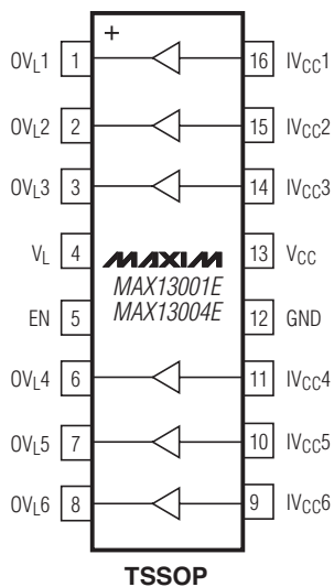
TSSOP
