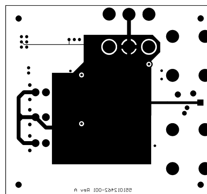
Bottom Layer
