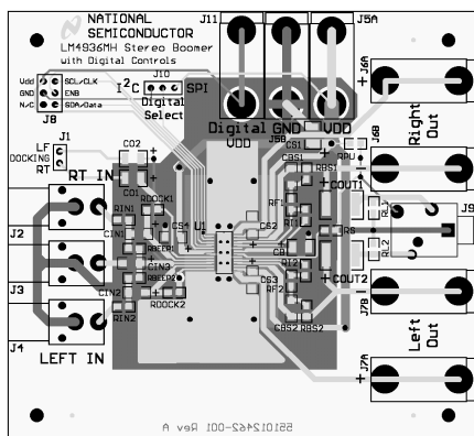
Top Layer
