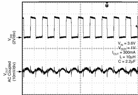
Ripple
