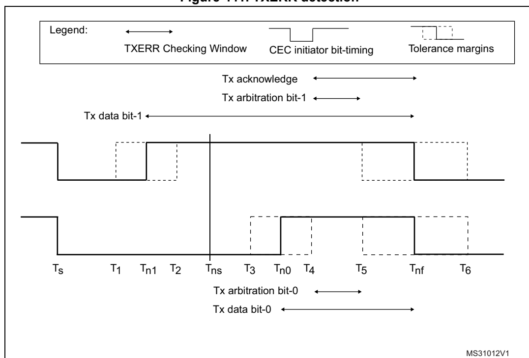
Figure 441. TXERR detection
