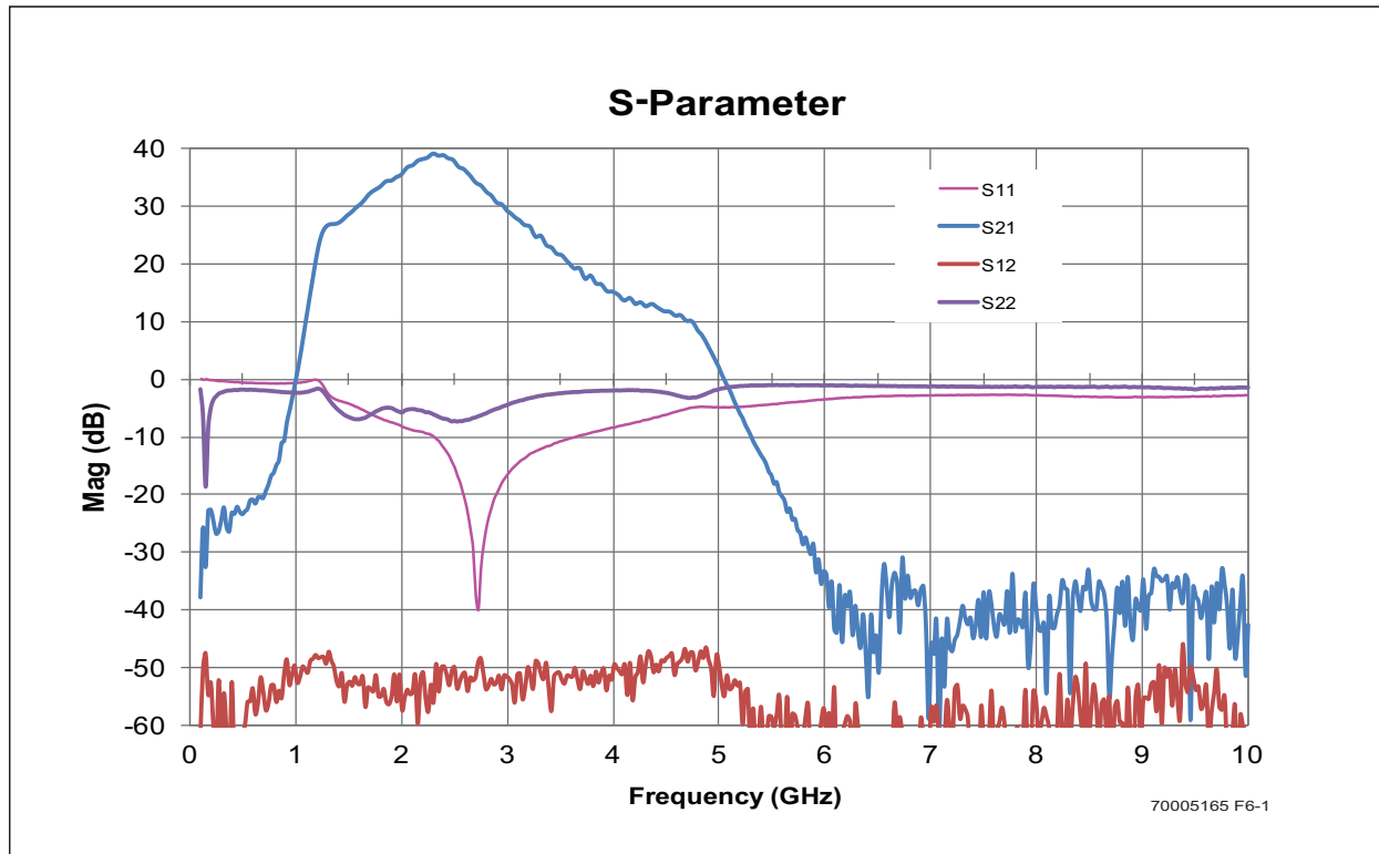
FIGURE 6-1: S-PARAMETER
