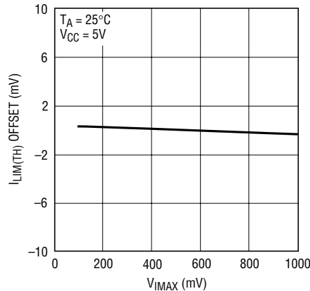
I_{LIM(TH)} Offset vs V_{IMAX}
