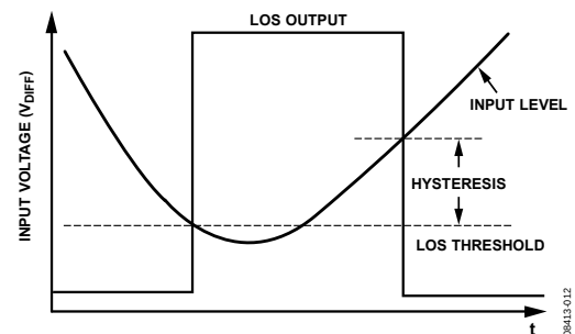
Figure 27. LOS Detector Hysteresis
