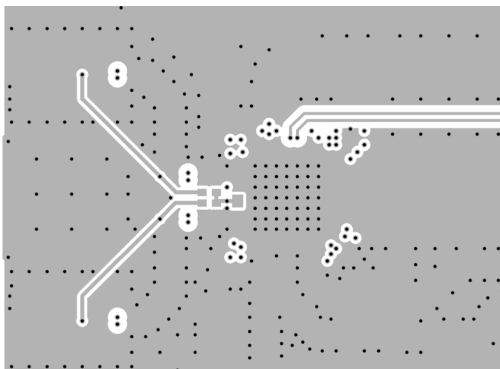
Bottom Layer
