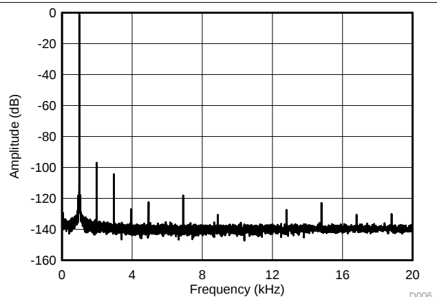
PCM1860-Q1, PCM1862-Q1, and PCM1864-Q1 Input = -1 dBFS at 1 kHz
