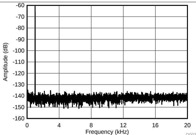
PCM1861-Q1, PCM1863-Q1, and PCM1865-Q1 Input = -60 dBFS at 1 kHz
