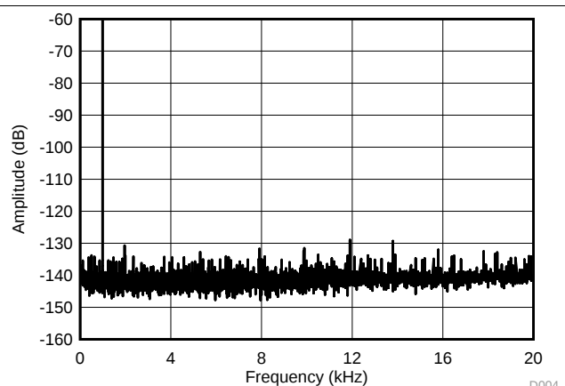
PCM1860-Q1, PCM1862-Q1, and PCM1864-Q1 Input = -60 dBFS at 1 kHz
