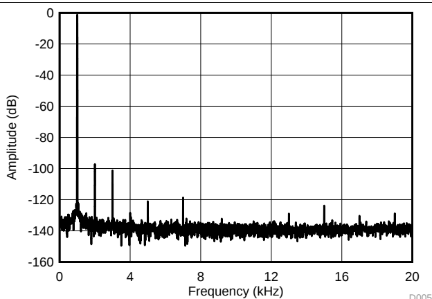
PCM1861-Q1, PCM1863-Q1, and PCM1865-Q1 Input = -1 dBFS at 1 kHz
