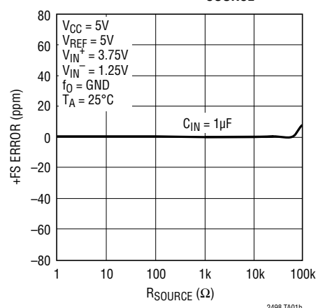
+FS Error vs R_{SOURCE}
