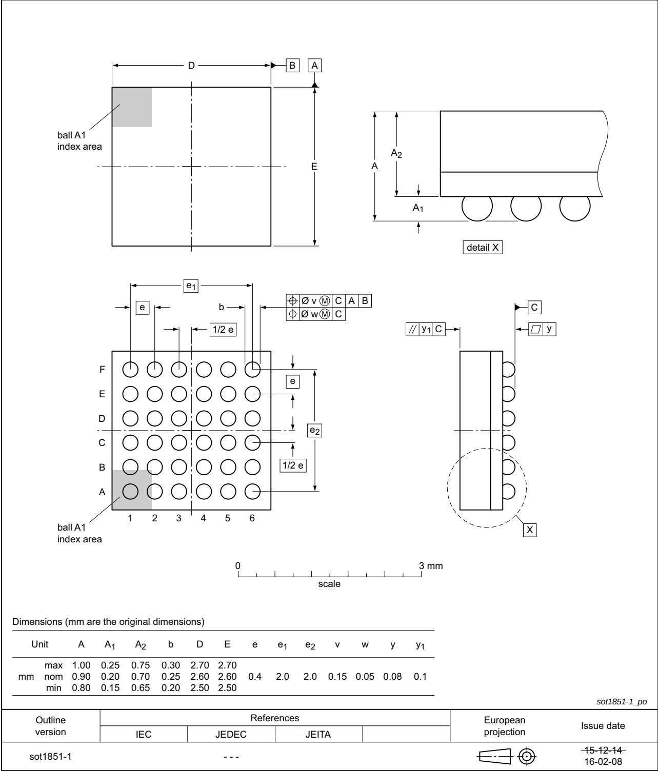
Fig 40. Package outline SOT1851-1 (VFBGA36)
