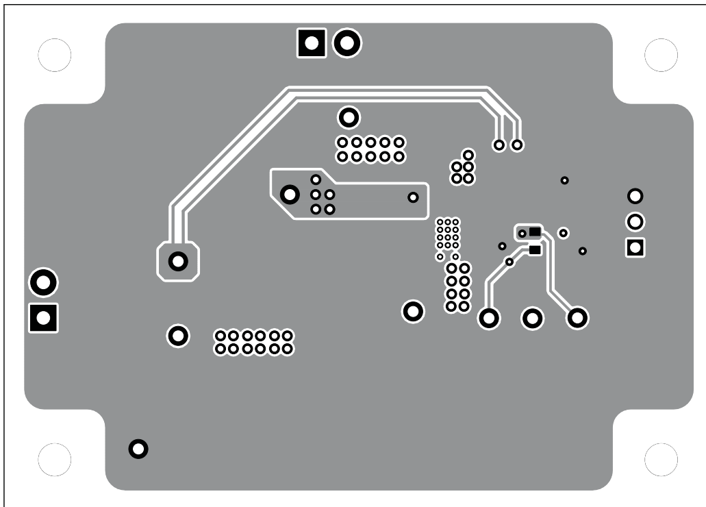
Figure 19. Bottom Layer
