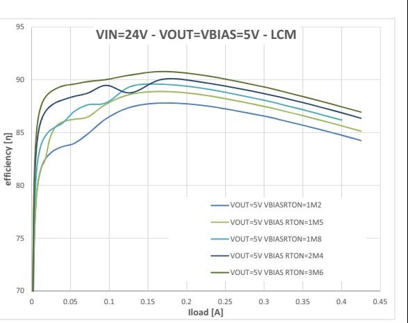
Figure 34. VIN 24 V - VOUT 5 V (linear scale)
