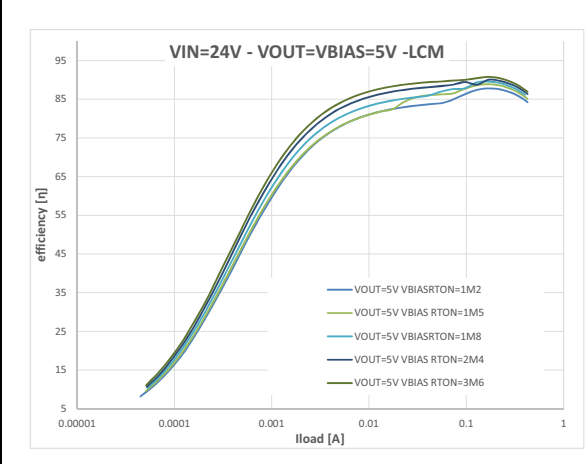
Figure 37. VIN 24 V - VOUT 5 V (log scale)
