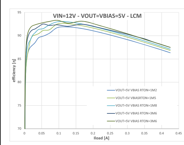
Figure 33. VIN 12 V - VOUT 5 V (linear scale)
