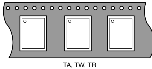
Figure 44. WLCSP 3-, 4-, 6-, 8-, 10-, & 12-Bump
