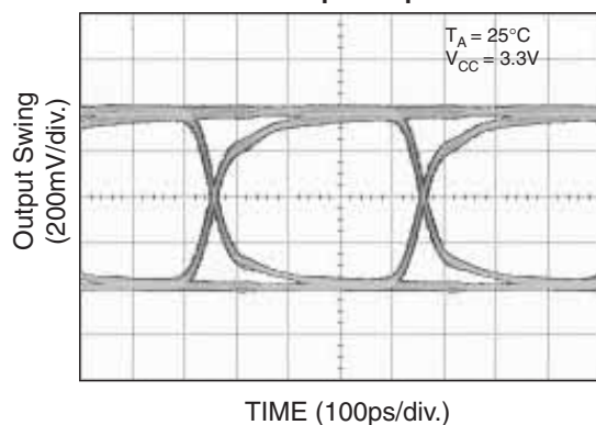
2.5Gbps Output
