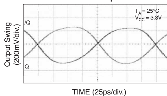
5GHz Output
