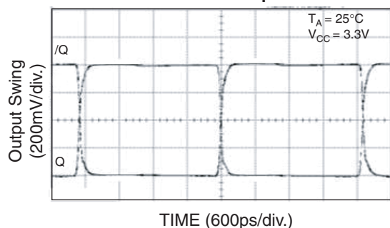
200MHz Output
