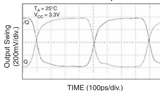
1.25GHz Output
