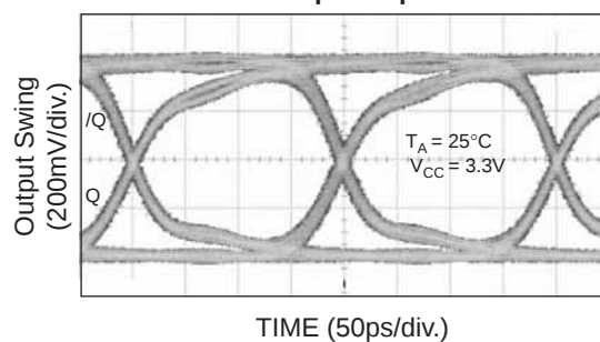
5Gbps Output
