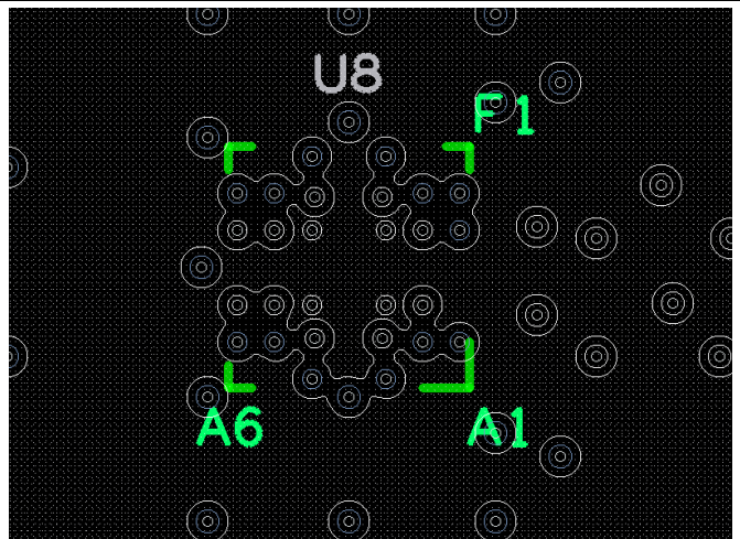
Figure 29. VDD Layer
