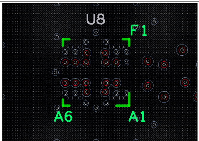
Figure 27. Layer 1 GND
