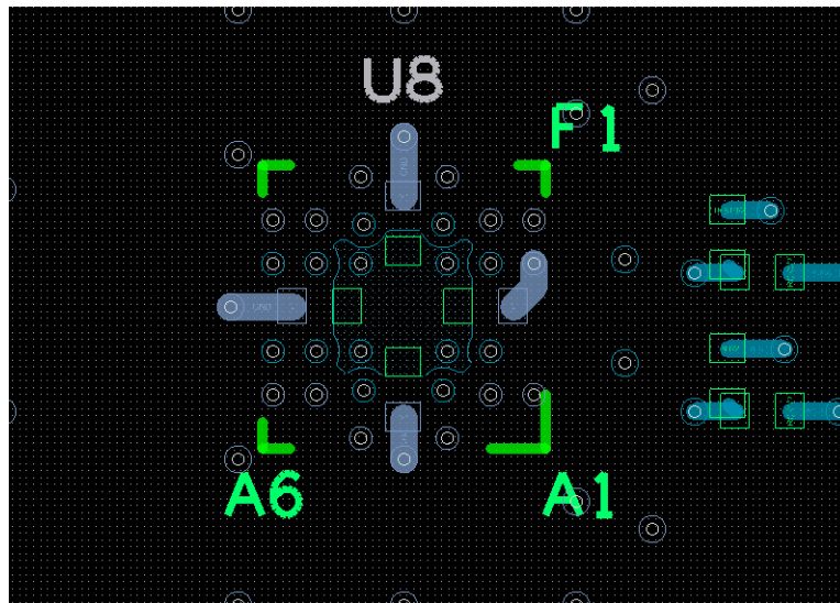
Figure 30. Bottom Layer
