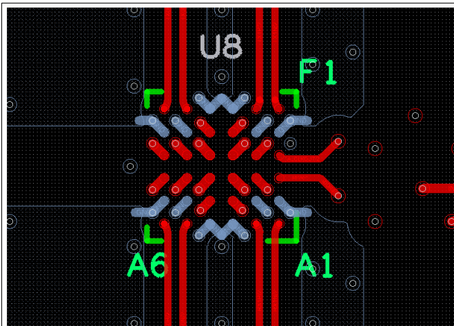
Figure 26. Top Layer
