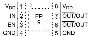
MCP14A0601/MCP14A0602 2 x 3 TDFN*
