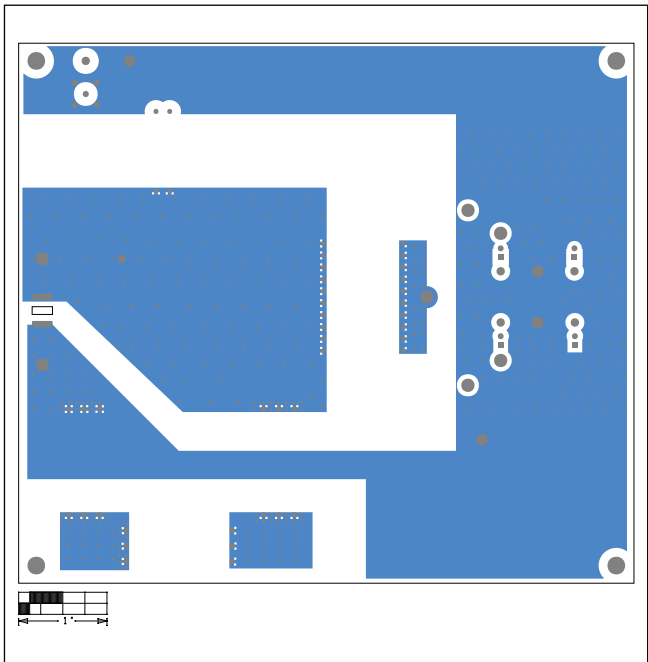
Bottom
