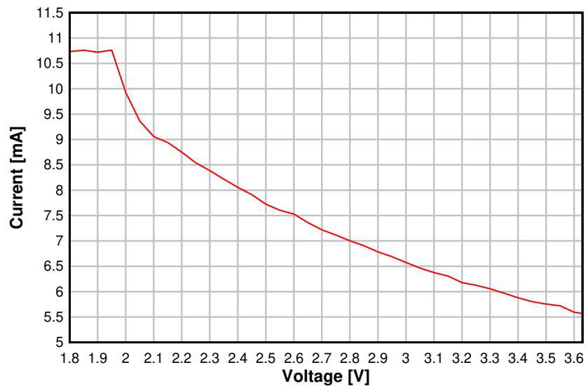
RX Current vs. VDD5 BLE 1 Mbps, 2.44 GHz
