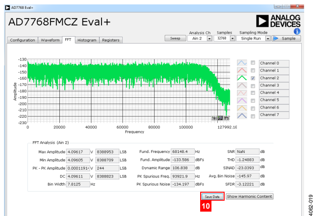
Figure 21. FFT Tab
