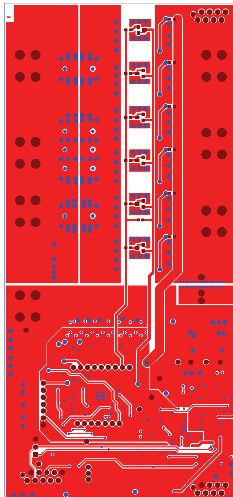
Figure 18. Bottom Layer
