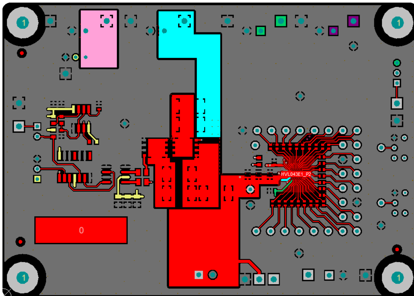
Figure 17. TS3DDR32611 EVM Top Layer
