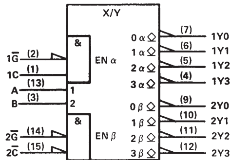
'156, 'LS156
