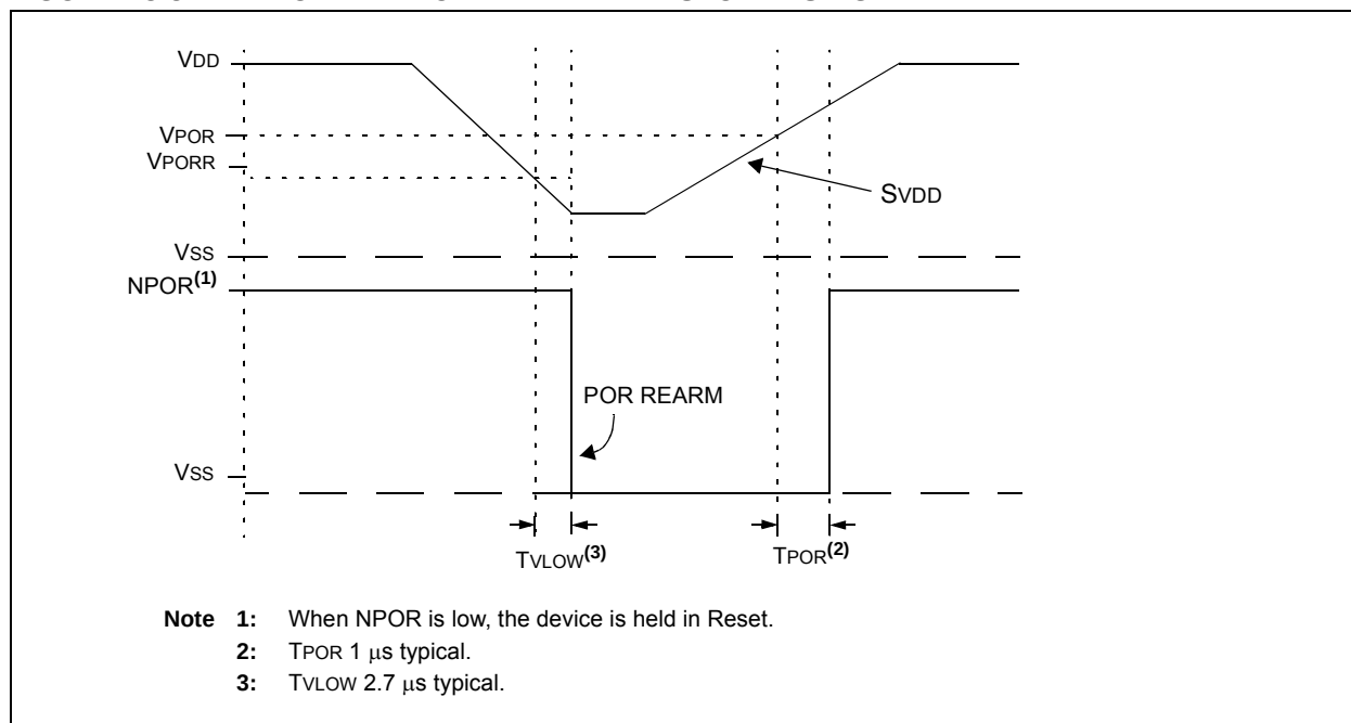
FIGURE 28-3: POR AND POR REARM WITH SLOW RISING V DD
