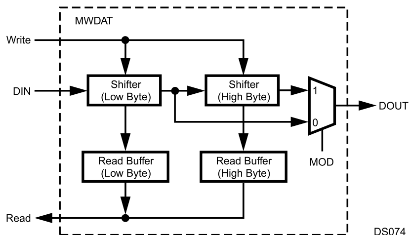
Figure 22-8. MWDAT Register
