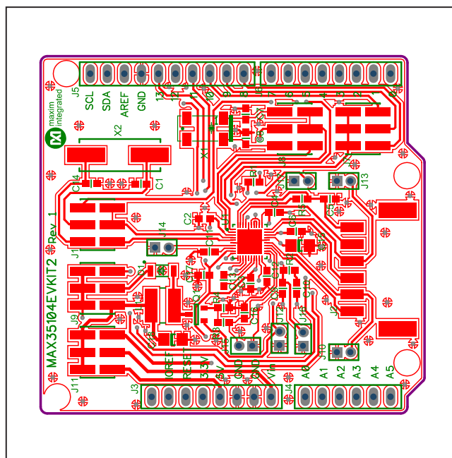
PCB Top
