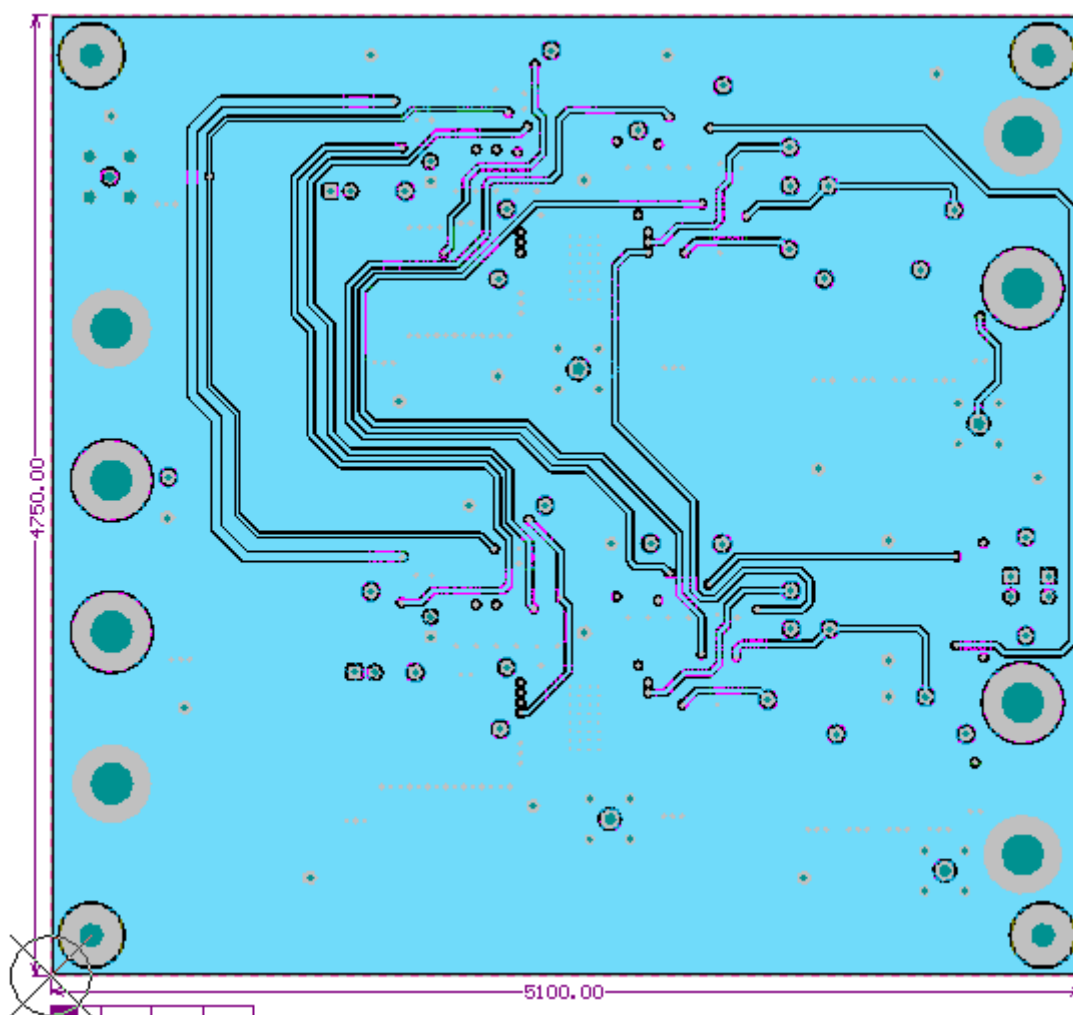
Figure 10. TPS50601ASPEVM Layer 3
