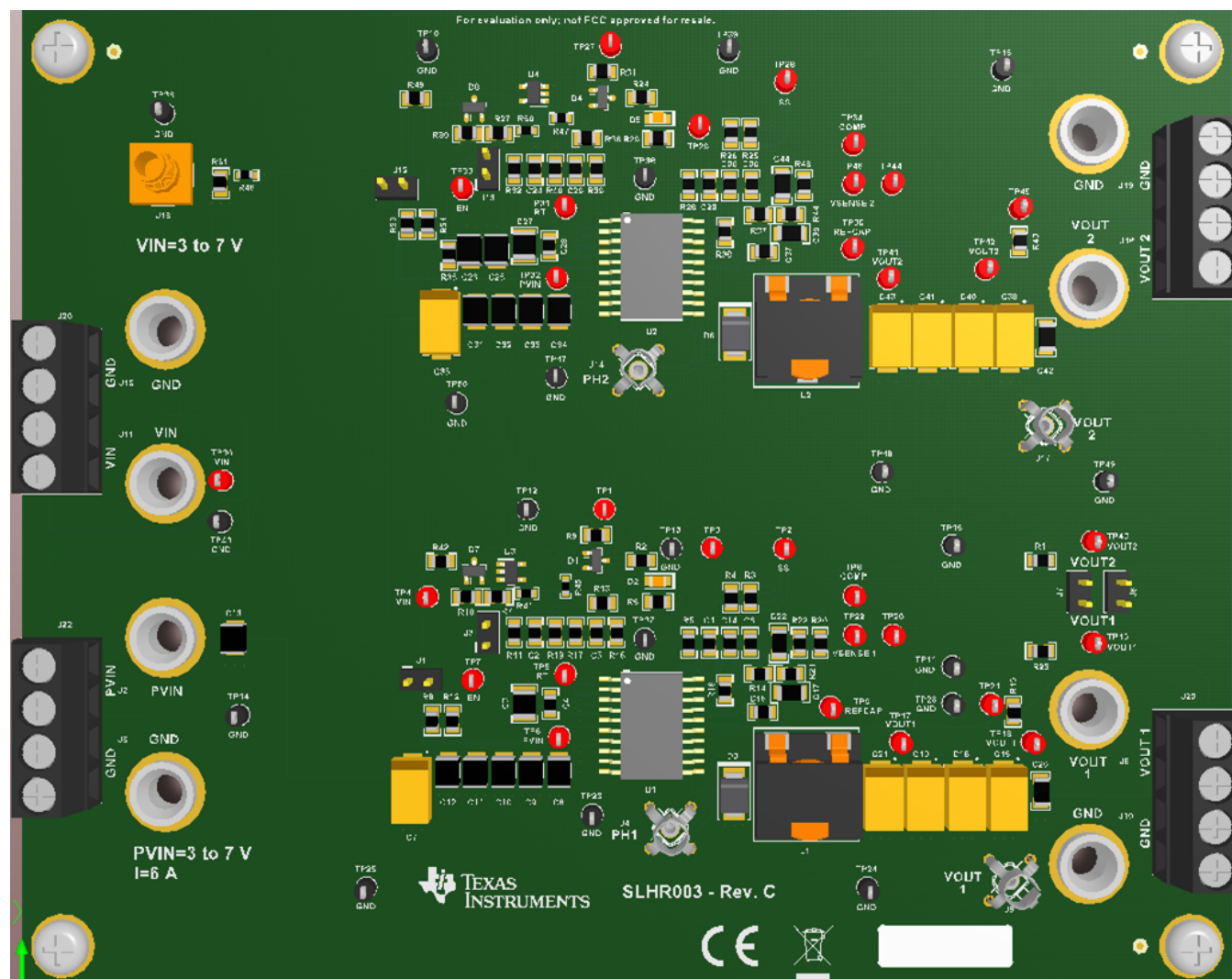
Figure 12. TPS50601ASPEVM Assembly
