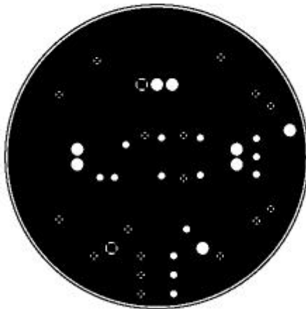
Layer 4: GND
