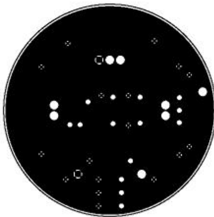
Layer 4: GND
