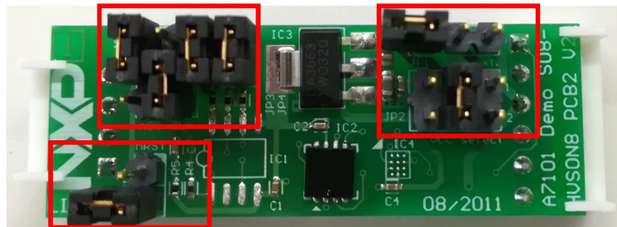
Fig 2. A71CH mini PCB OM3710/A71CHPCB
