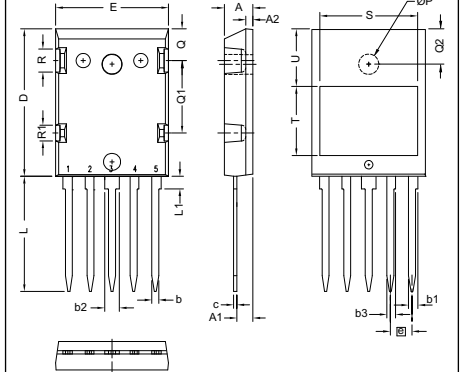
XO23 ISO264™ Weight = 6.5 g
