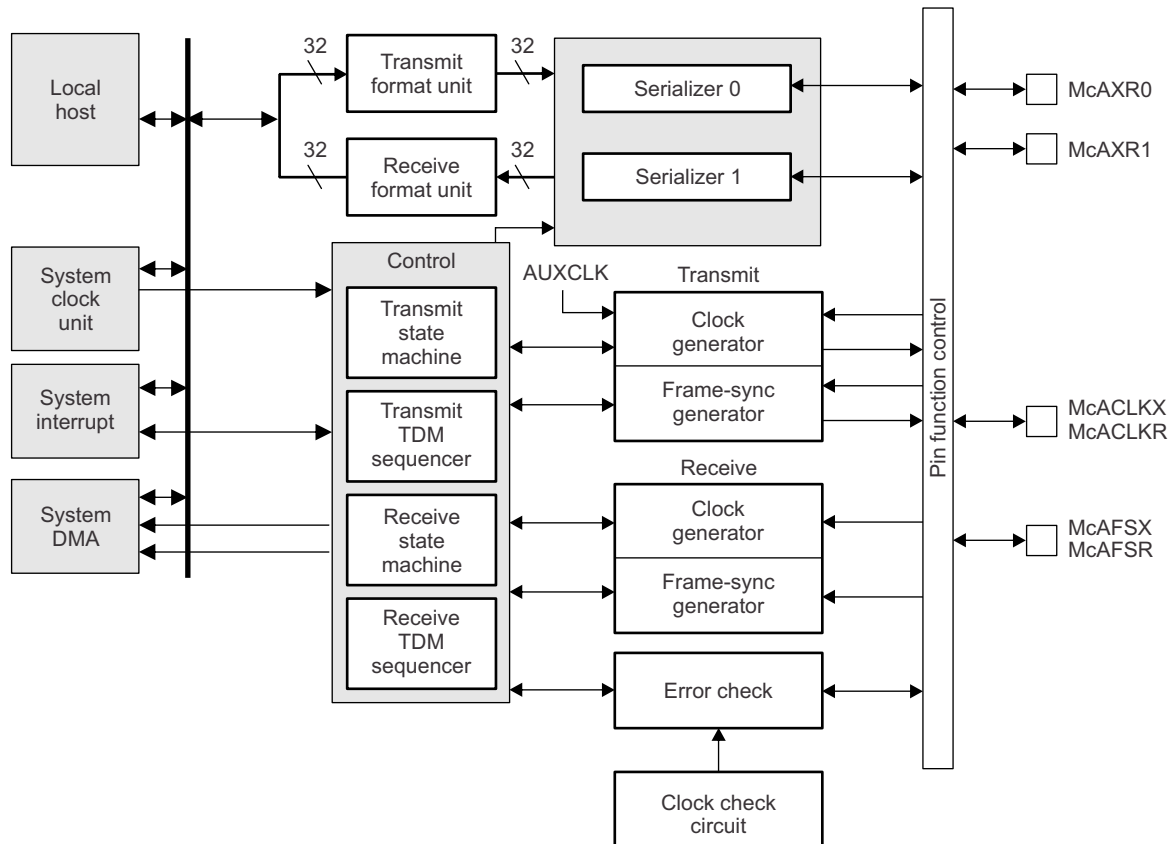
Figure 12-2. MCASP Module
