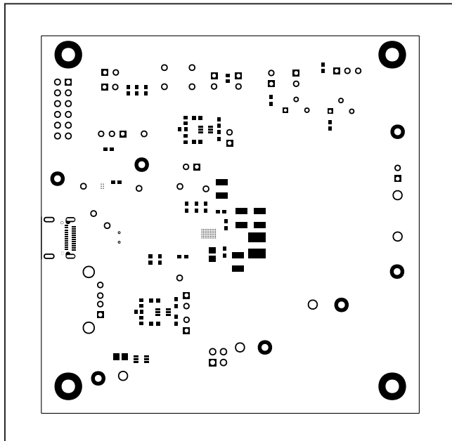
MAX14748 EV Kit—Mask Top
