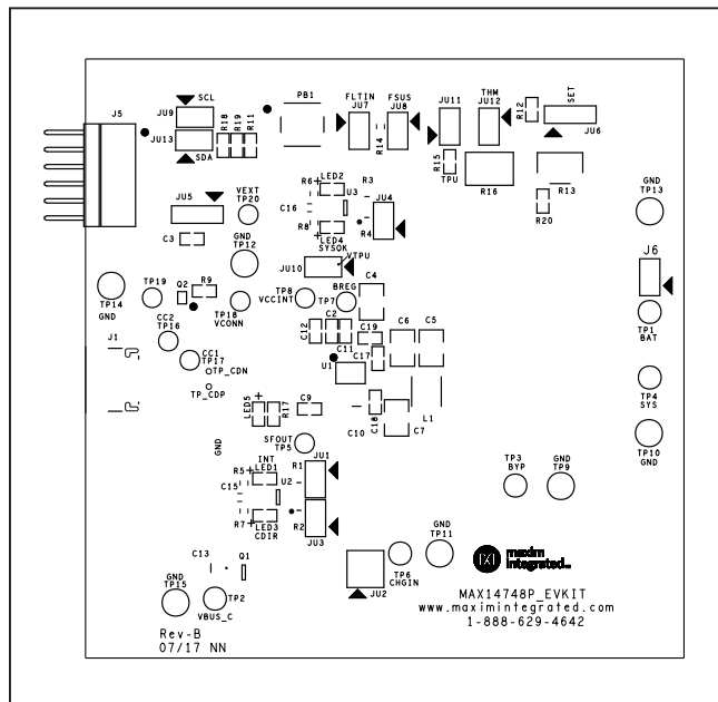
MAX14748 EV Kit—Silk Top
