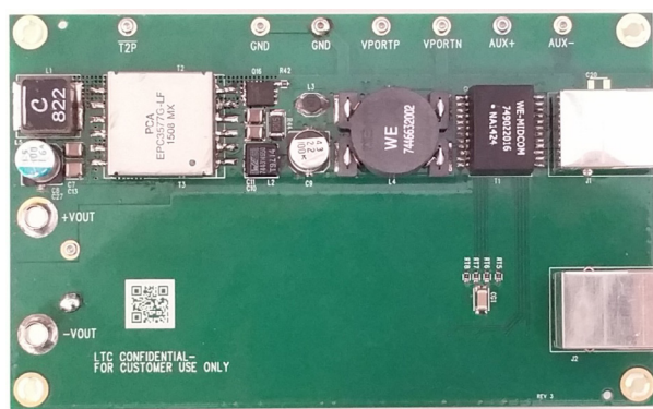
Bottom Side
