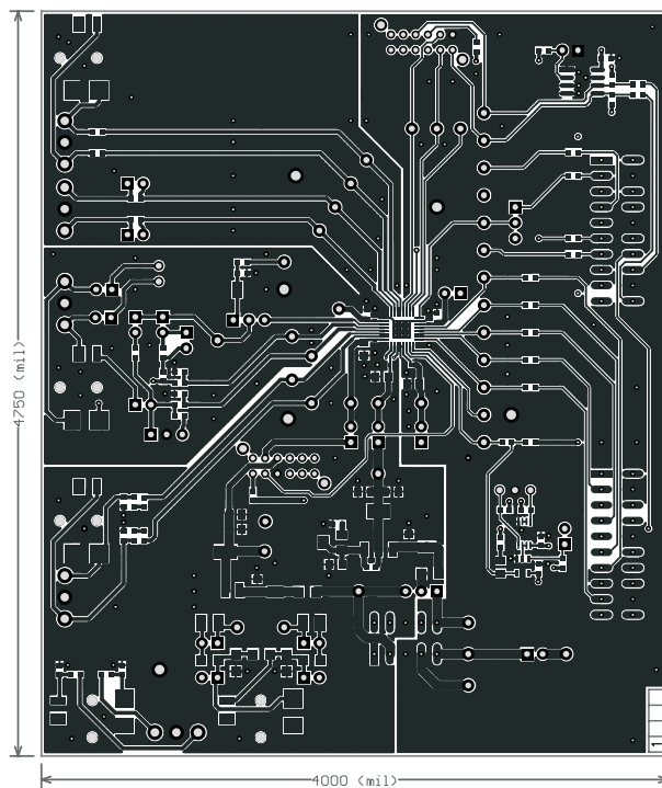
Figure 20. Top Layer
