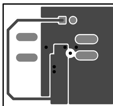
Figure 33. Bottom Layer
