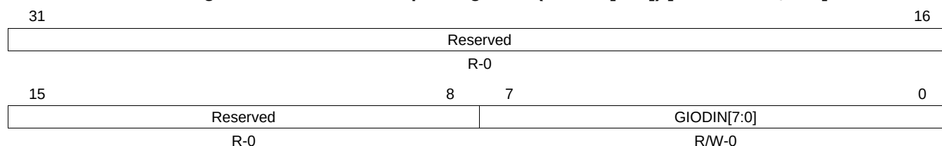
Figure 23-18. GIO Data Input Registers (GIODIN[A-B]) [offset = 38h, 58h]
