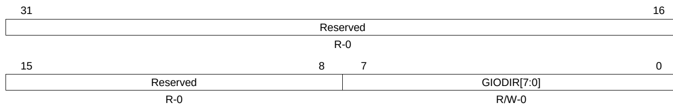
Figure 23-17. GIO Data Direction Registers (GIODIR[A-B]) [offset = 34h, 54h]
