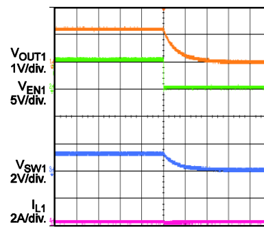
EN Down without Load (CH1)
