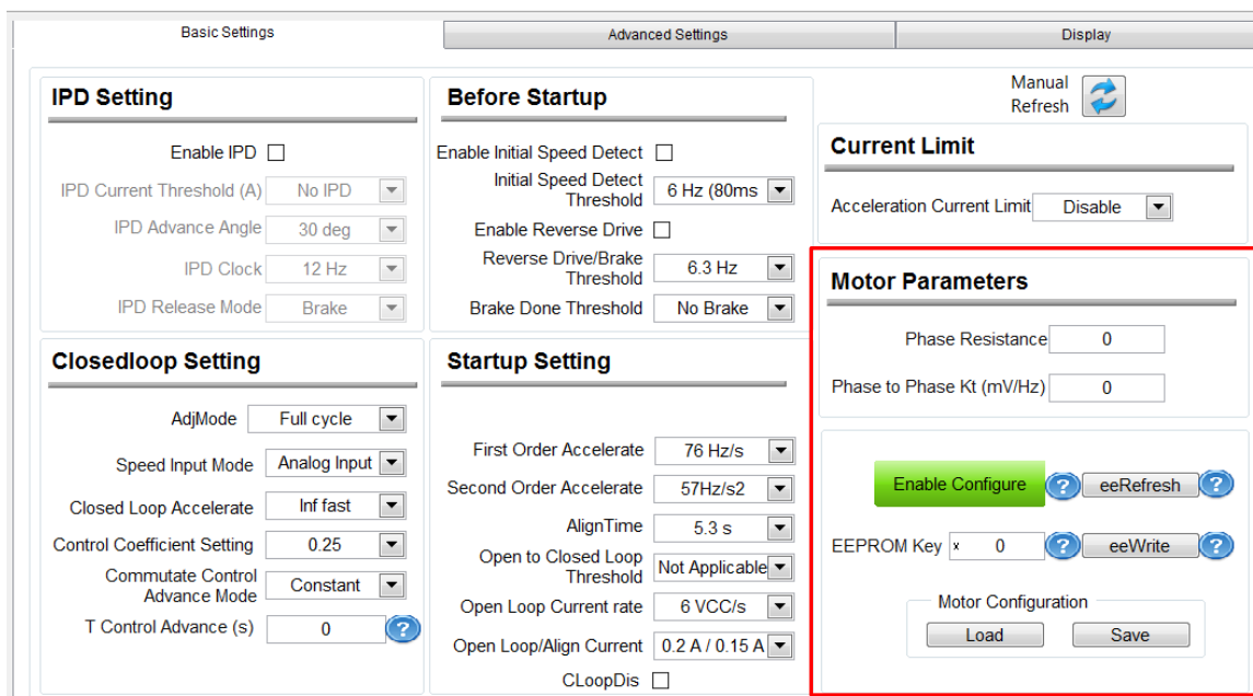
Figure 4. Motor Parameters
