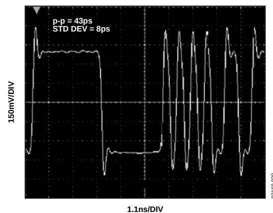
Figure 20. Response, 3.2 Gbps, 32-Bit Pattern 1111 1111 0000 0000 0101 0101 0011 0011
