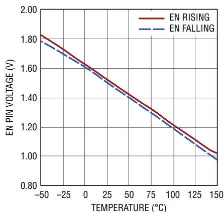
Enable Threshold
