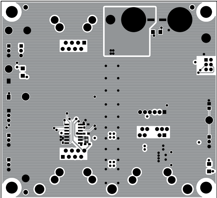
Layer 1
