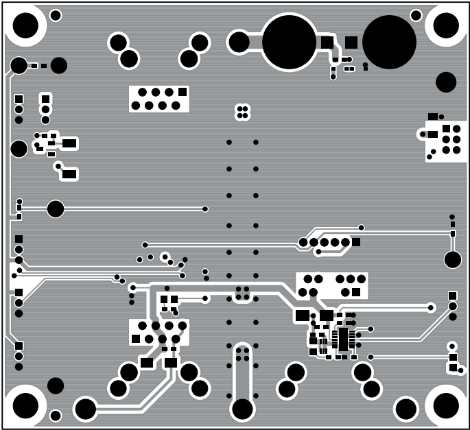
Layer 4
