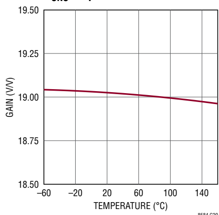
V_{SNS} Amplifier Gain
