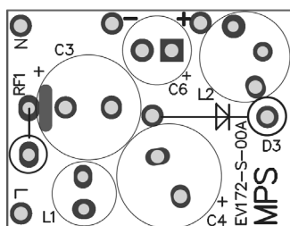
Top layer
