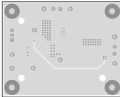
Figure 18. Bottom Layer
