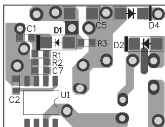
Bottom layer
