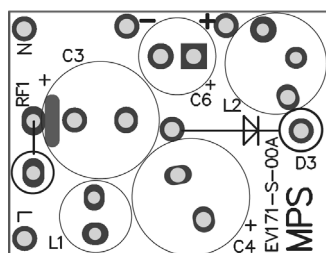
Top layer
