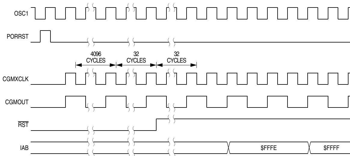
Figure 15-7. POR Recovery
