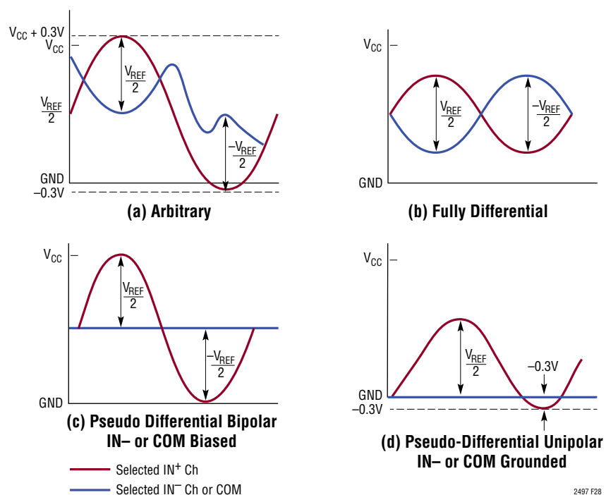
Figure 28. Input Range
