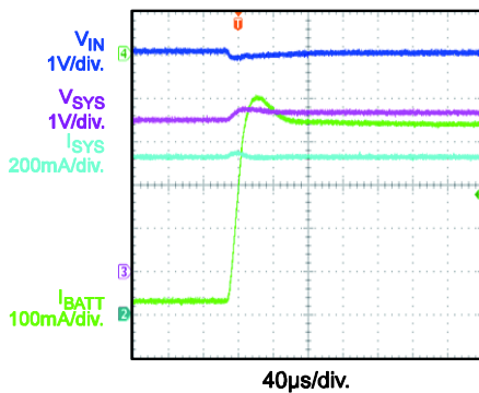
EN On @ Supplement Mode
