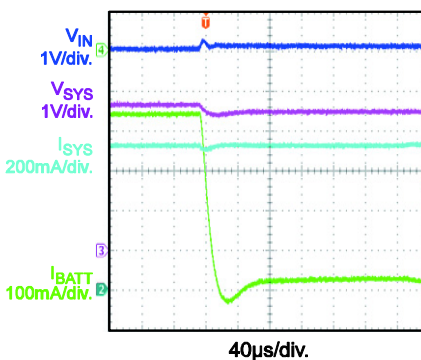
EN Off @ Supplement Mode
