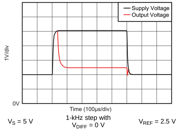
图 22. Brownout Recovery
